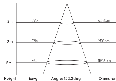
22W/ UGR<25/ 130LM/W
