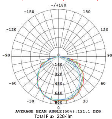
18W/ UGR<35/ 130LM/W
