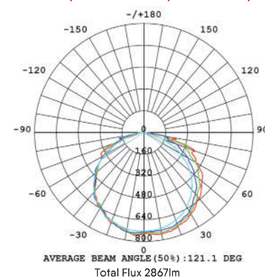
22W/ UGR<25/ 130LM/W
