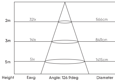
18W/ UGR<35/ 130LM/W
