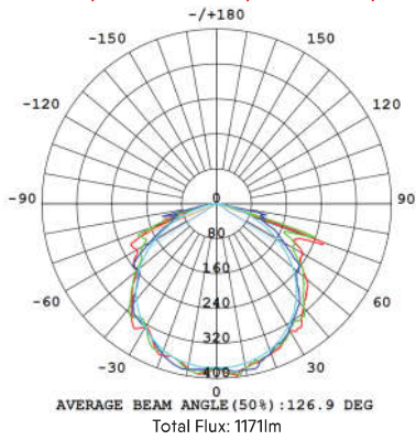
9W/ UGR<30/ 130LM/W
