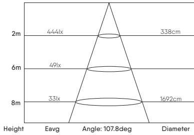
TI/185W/UGR<43/130LM/W
