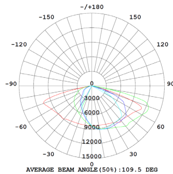
TI/240W/UGR<41/130LM/W
