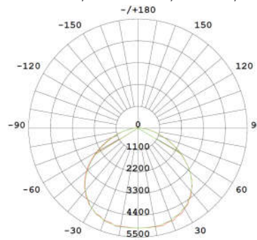
150W/UGR<23/111LM/W
